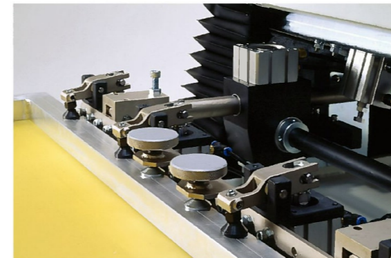
スピーディーな版固定、エア断でも版を保持
