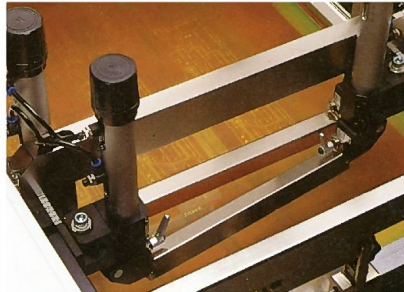
ななめスキージ(タイプA)
