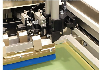
ななめスキージ(タイプB)
